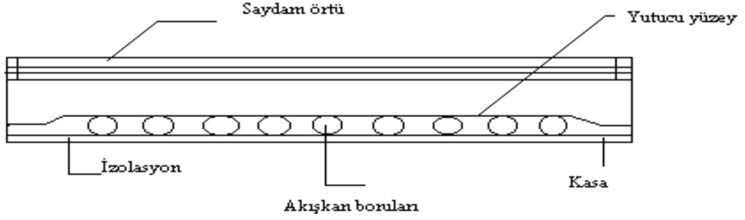
Şekil 1.2. Düz Toplayıcı Yapısının Yandan Görünüşü
